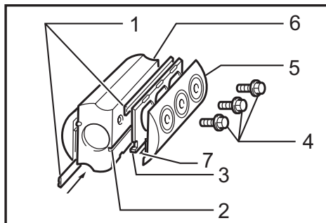
► 1. Cuchilla del cepillo 2. Ranura 3. Placa de fijación 4. Pernos de cabeza hexagonal para brida 5. Cubierta del tambor 6. Tambor 7. Placa de ajuste
