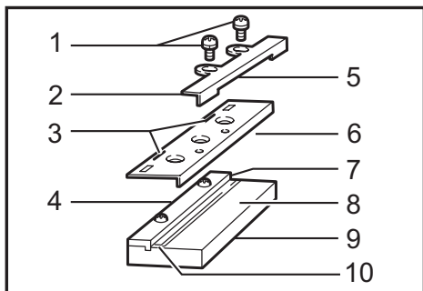
► 1. Tornillo de cabeza grande 2. Placa de ajuste 3. Juntas de posicionamiento de la cuchilla del cepillo 4. Placa calibradora 5. Pie de la placa de ajuste 6. Placa de fijación 7. Cara interna de la placa calibradora 8. Base del calibre 9. Lado trasero de la base del calibrador 10. Cuchilla del cepillo
